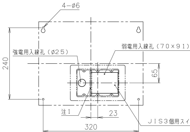
取付寸法図
