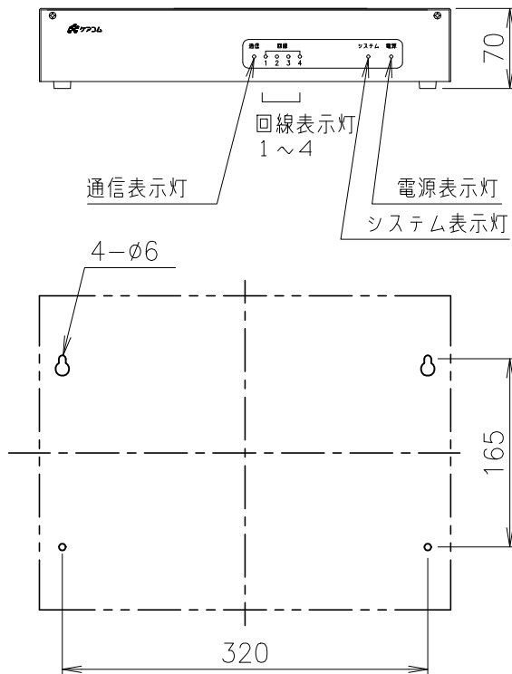
取付寸法図
