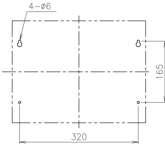
取付寸法図
