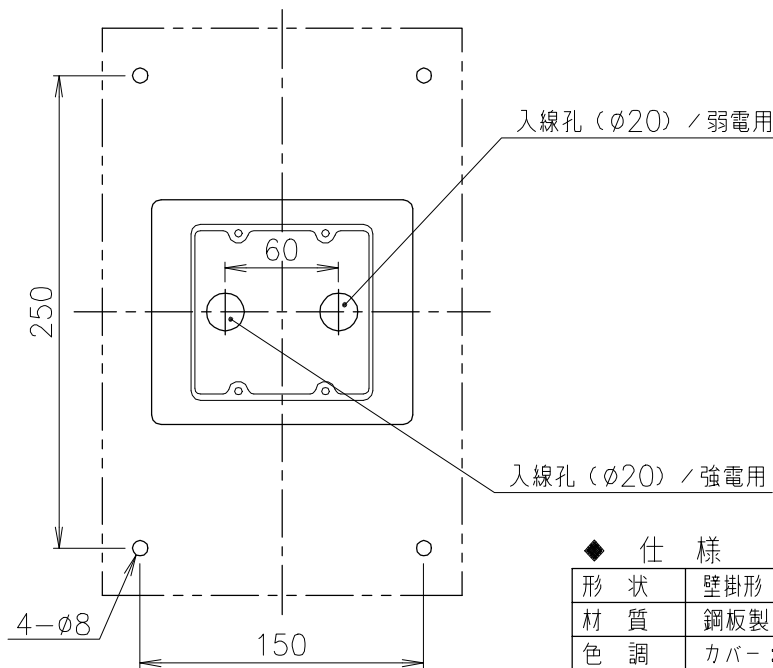
取付寸法図
