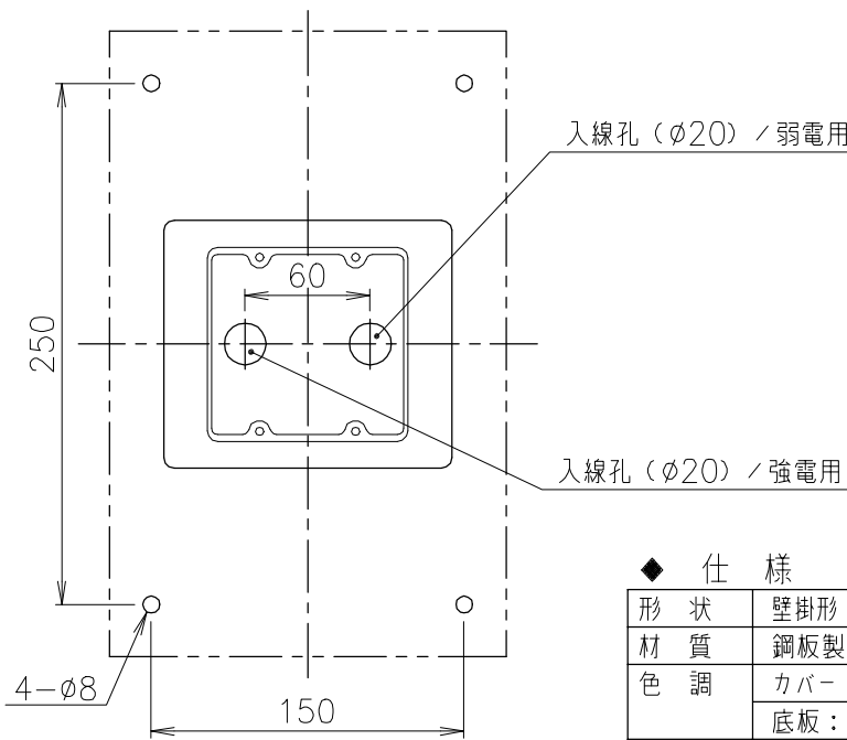
取付寸法図
