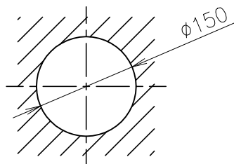
天井吸音材穴加工寸法図
