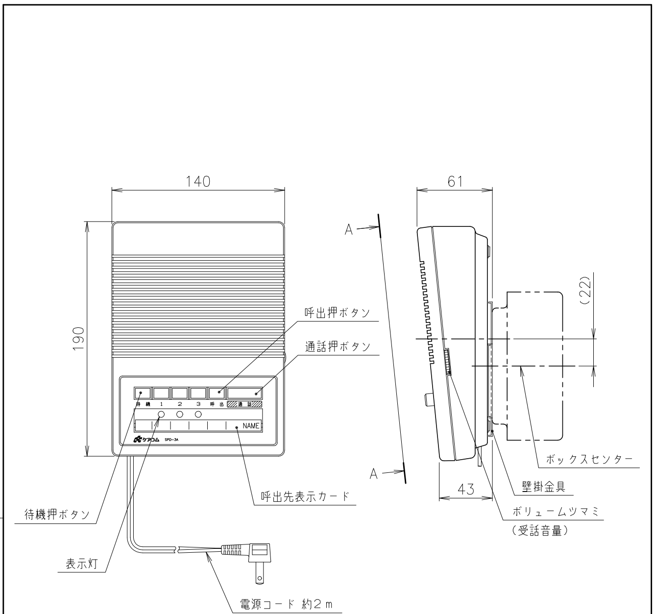
A - A 矢視
