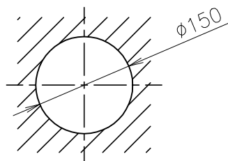
天井吸音材穴加工寸法図
