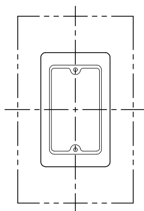
取付寸法図
