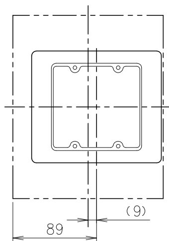
取付寸法図
