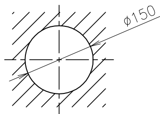
天井吸音材穴加工寸法図
