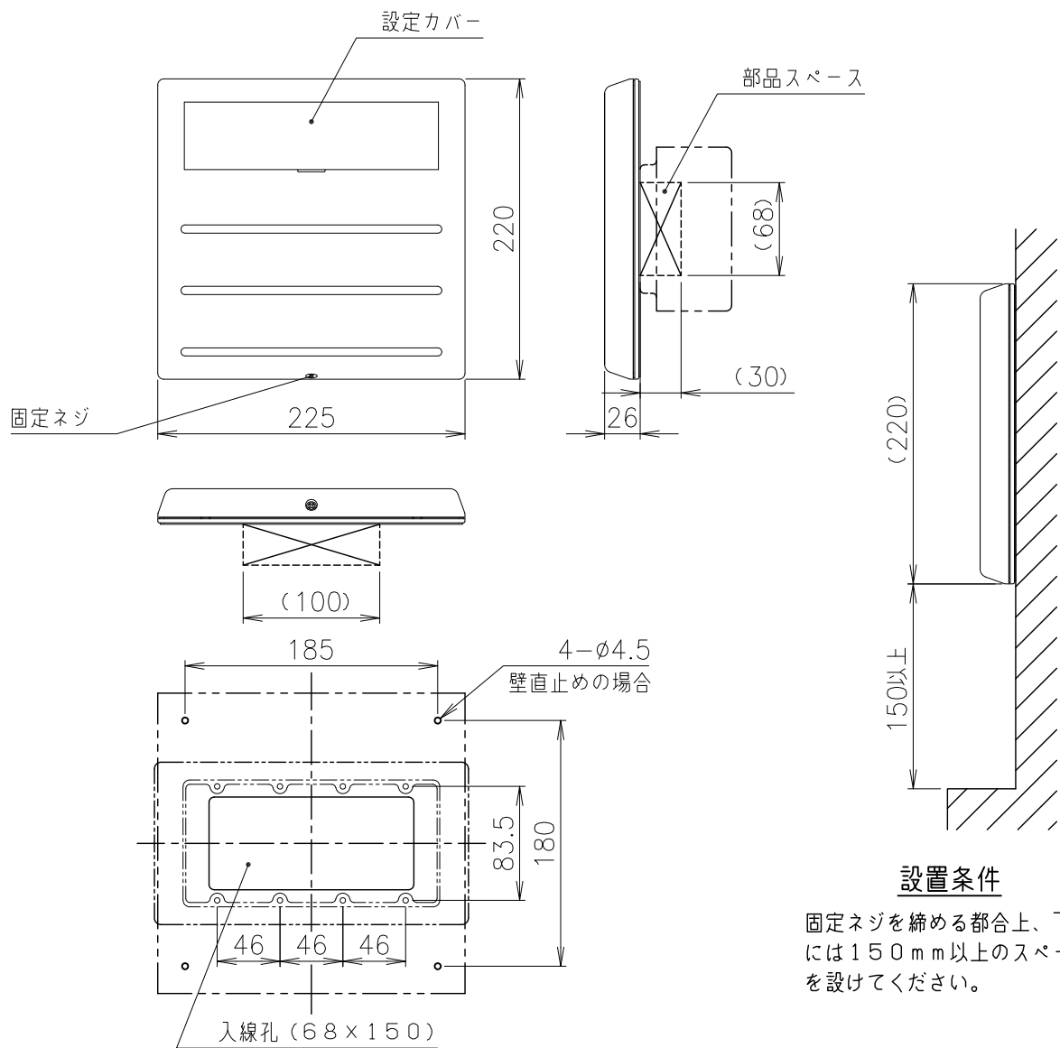
取付寸法図
