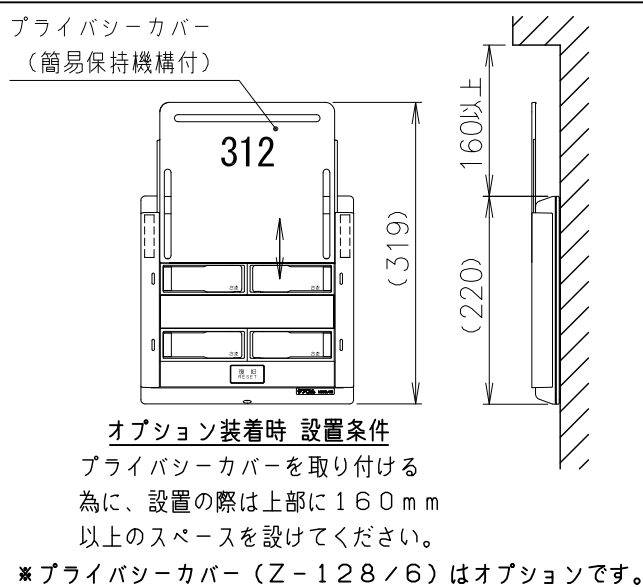
取付寸法図
