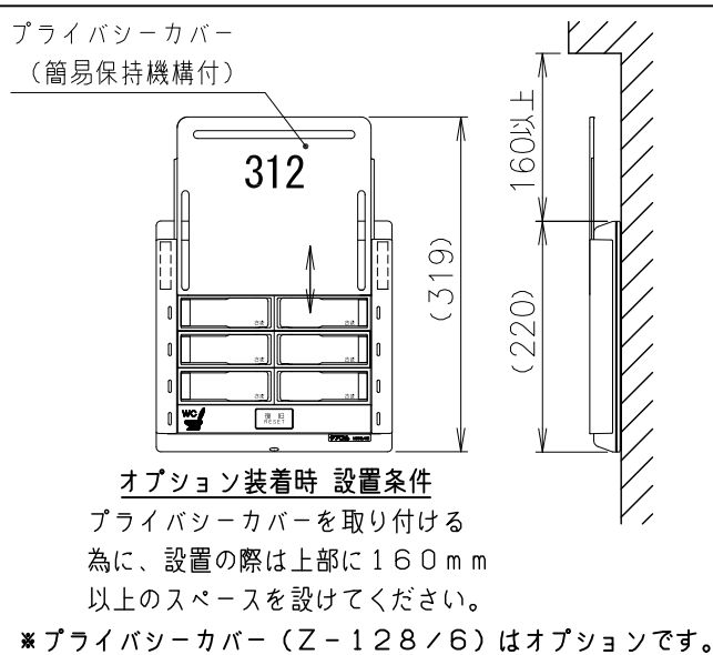
取付寸法図
