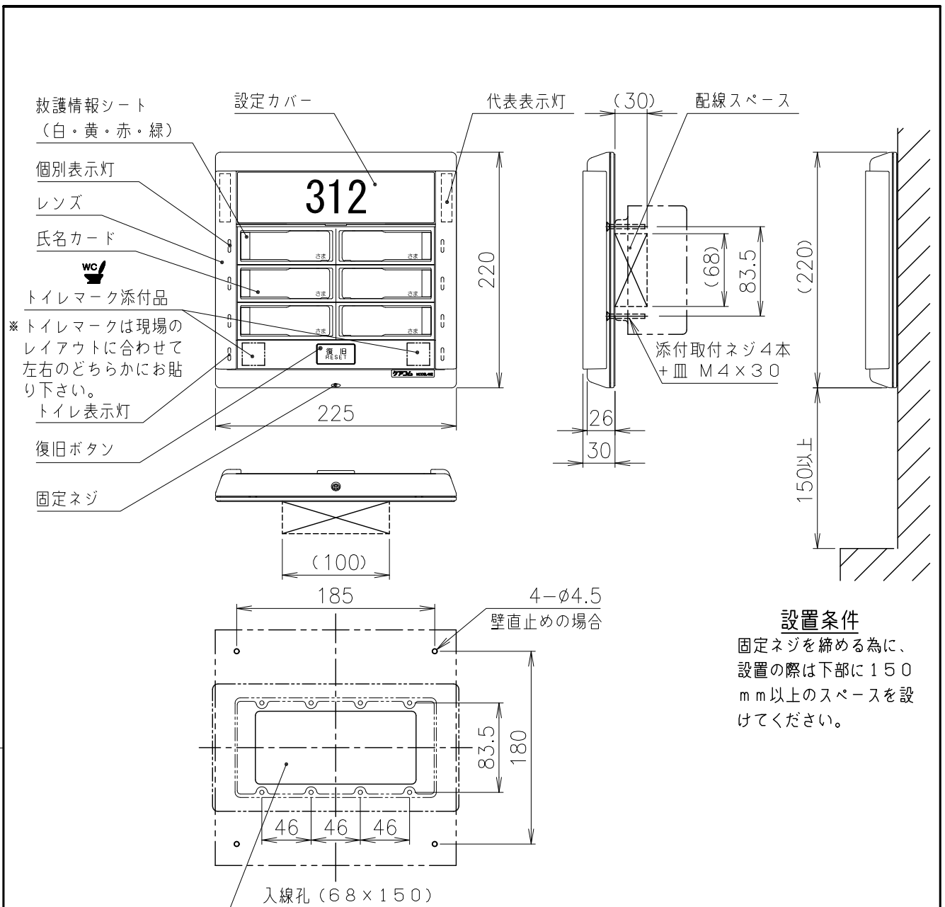
取付寸法図
