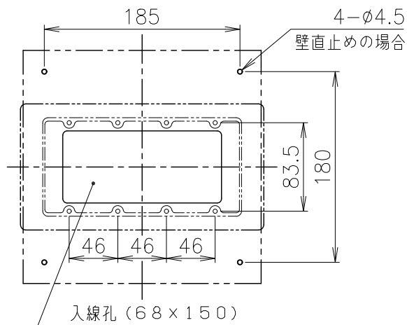
取付寸法図
